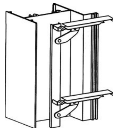
ISOMÉTRICO CELOSIA DE LUJO G-28 DE 2" CLG028
